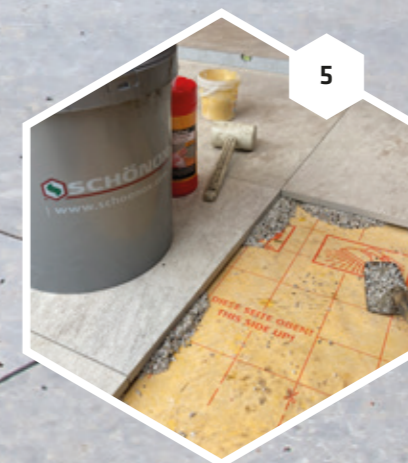
5 Mittels Gummihammer und Wasserwaage die Fliesen oder Platten ausrichten.
