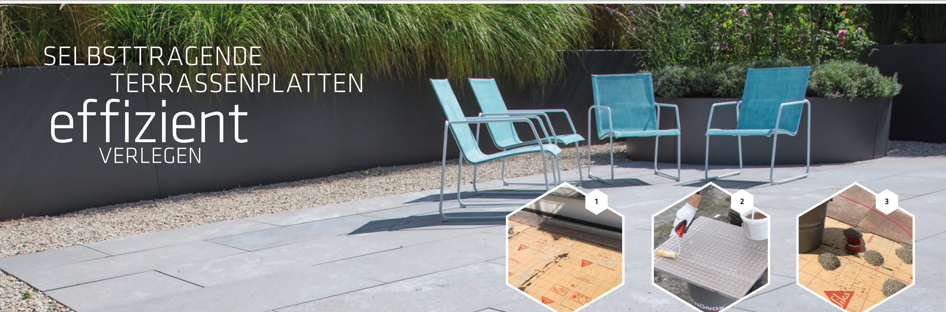
1 Abdichtung mit dem Dichtkleber SCHÖNOX iFIX® und der Abdichtungsbahn SCHÖNOX AB 30/ AB 10.
