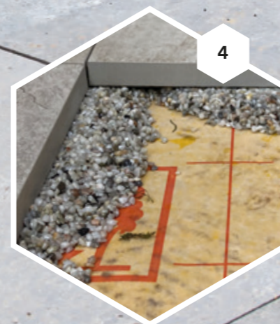
4 Die Fliesen oder Platten in die Batzen einlegen.
