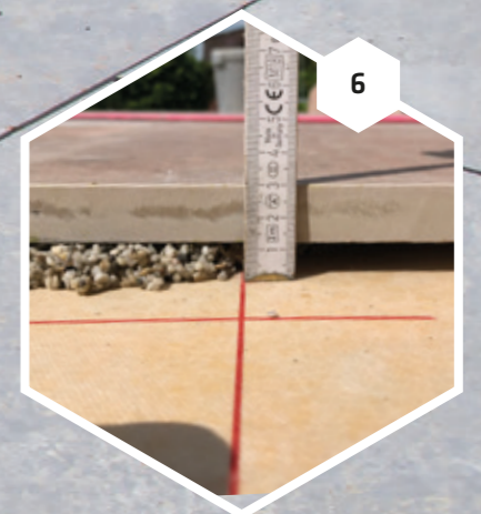
6 Bei Abschlüssen die Plattenränder mit SCHÖNOX EP DRAIN unterfütern.
