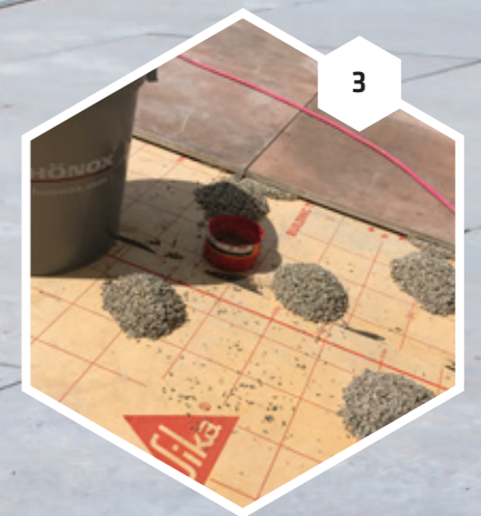
3 SCHÖNOX EP DRAIN gemischt mit SCHÖNOX MONOKORN in Batzenform auf den Boden aufbringen.*
