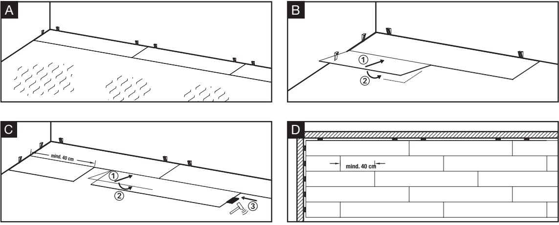
①= längsseitig Feder zusammenfügen, ②= einwinkeln, ③= stirnseitig verbinden
